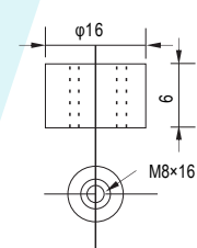
КЛЕММ Т19
